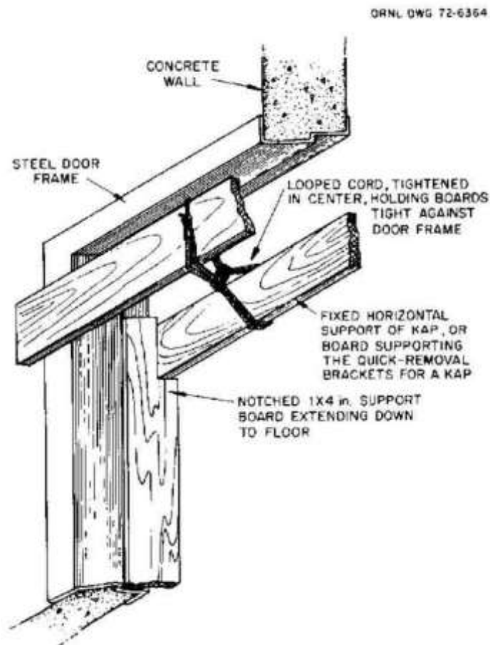
Fig. 28. Steel door frame. ORNL DWG 72-6564
